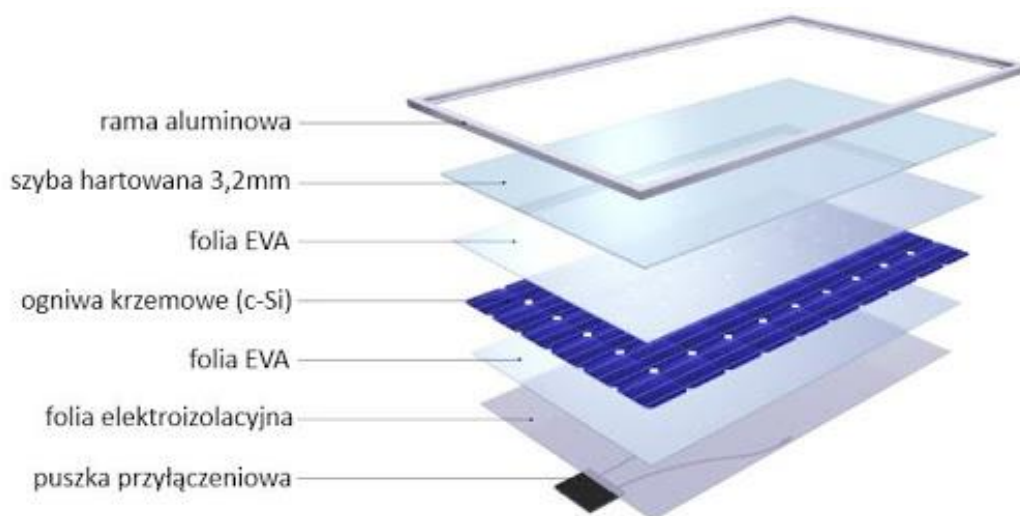
Rycina 7. Przekrój poetyczny modułu fotowoltaicznego.
